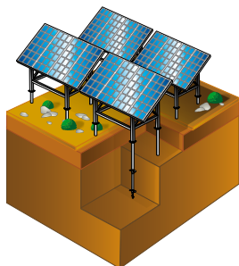
Maintien de panneau photovoltaïque
